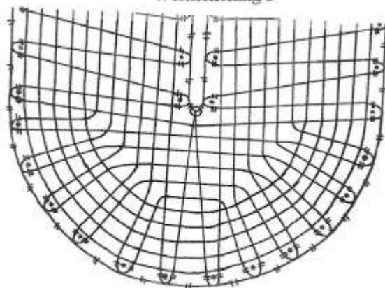
Werktekening 2
